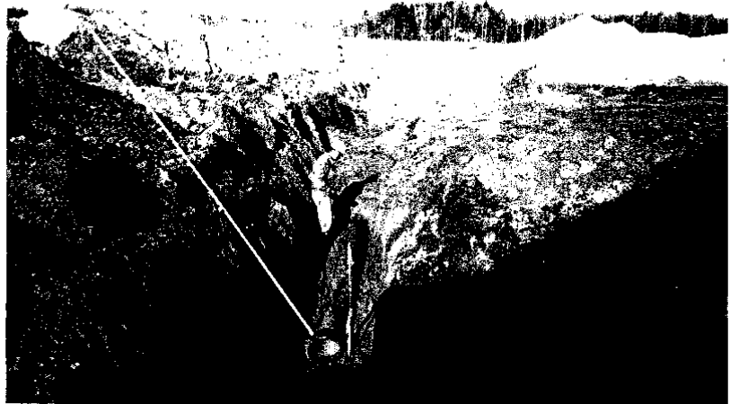
42 pav. Klojama kaupo 1-os sekcijos filtrato drenažo linija d-315.
