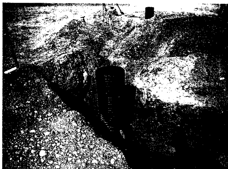
16 pav. Lietaus nuotekų tinklai Rokiskio žaliųjų atliekų kompostavimo aikštelėje
