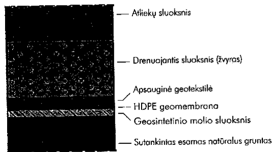
Sąvartyno dugno konstrukcija
