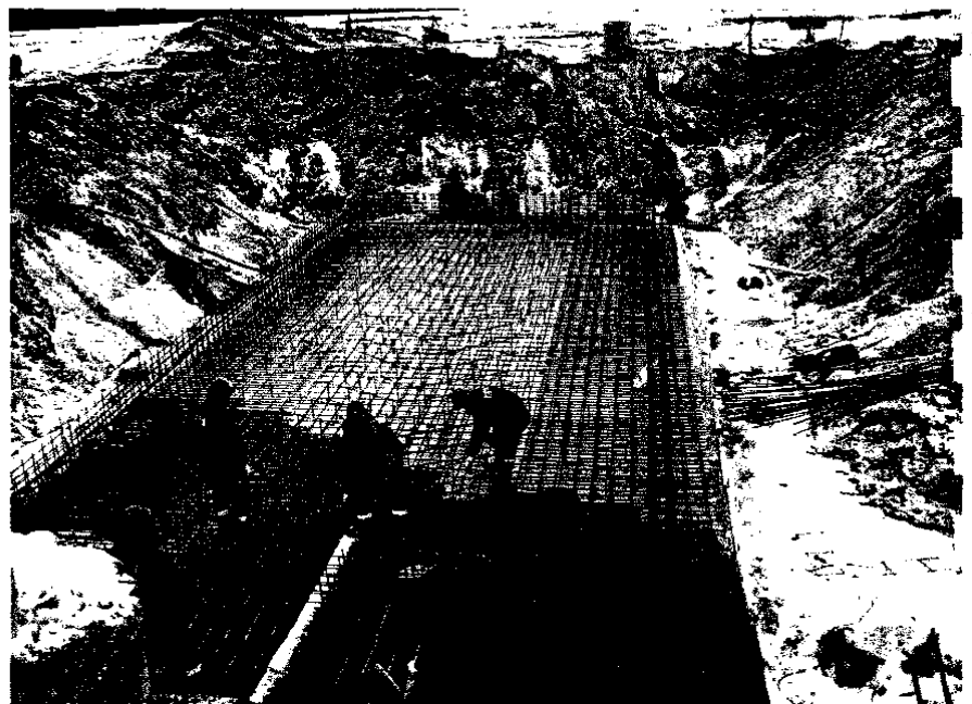
81 pav. Armatūros rėšimas ir betonavimas rezervuare.
