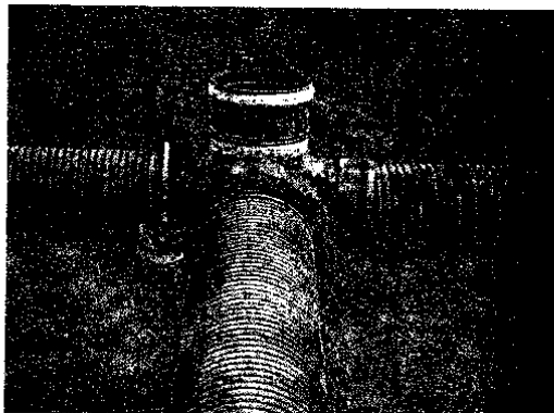
56 pav. Montuojamas šulinys SH-06, įjungiamosios linijos iš 500 ir 400 ultra PVC vamzdžių
