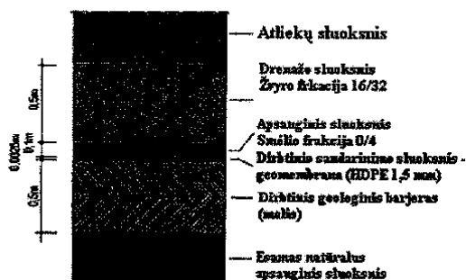
101 pav. Aukštrakių sąvartyno dugno konstrukcija
