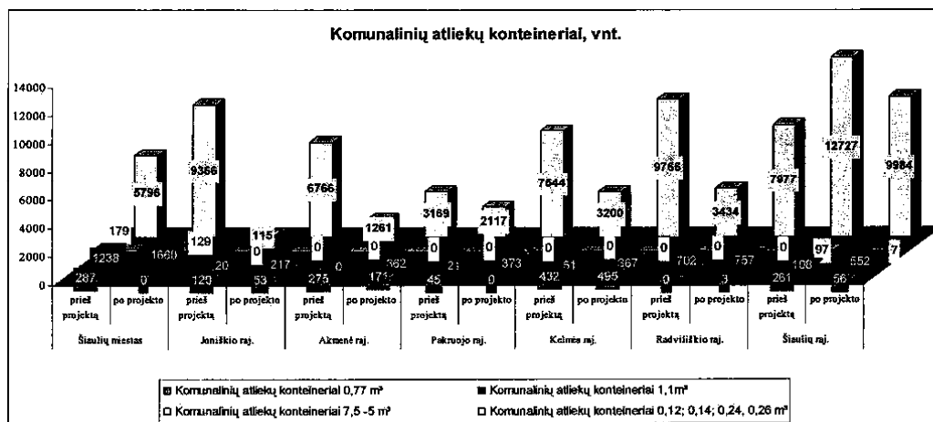
98 pav. Komunalinių atliekų konteineriai
